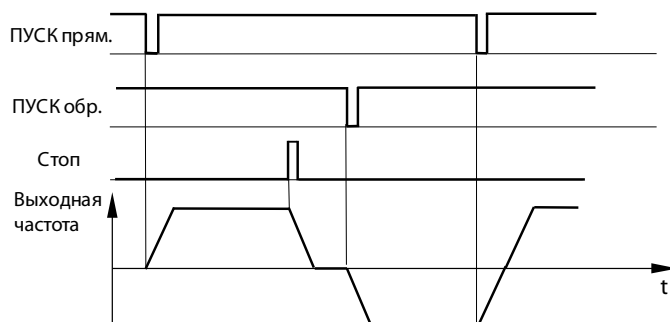
Рис.2б Трёхпроводное управление P5.00=2
