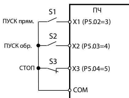
Рис.2а Трёхпроводное управление 1 P0.02=1, P5.00=2
