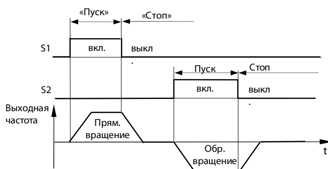
Рис.1б Двухпроводное управление 1 P5.00=0
